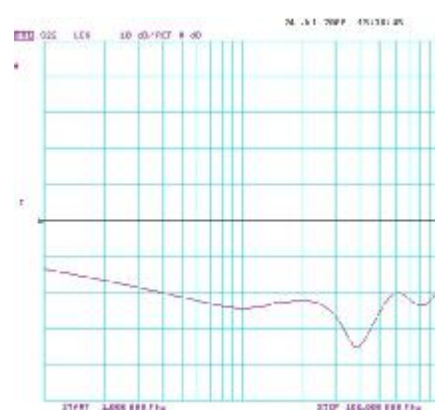
图 9 S22
